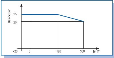
Grafik 1 : Basınç - sıcaklık ilişkisi Nota : 1 bar = 10 5 N/m 2 = 100kPa
